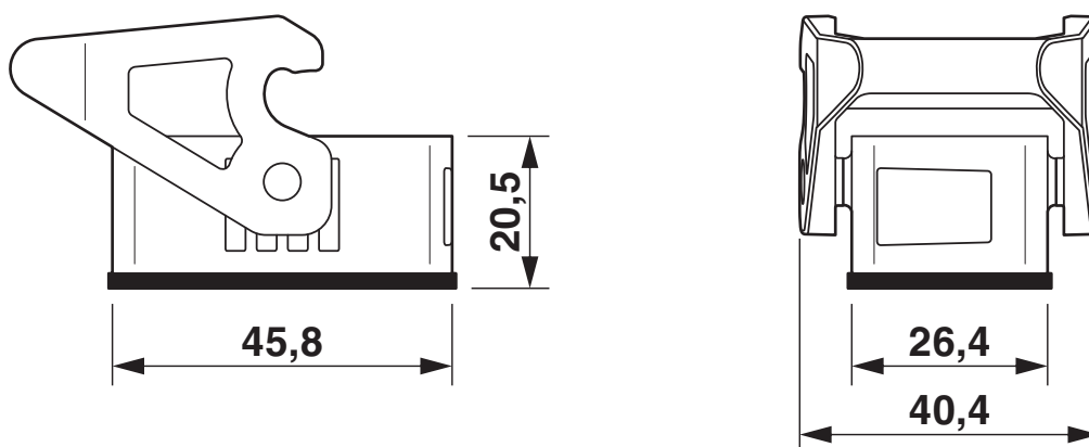
Rysunek wymiarowy
