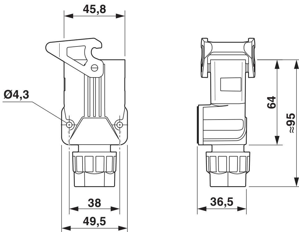
Rysunek wymiarowy
