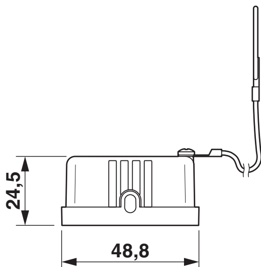
Rysunek wymiarowy
