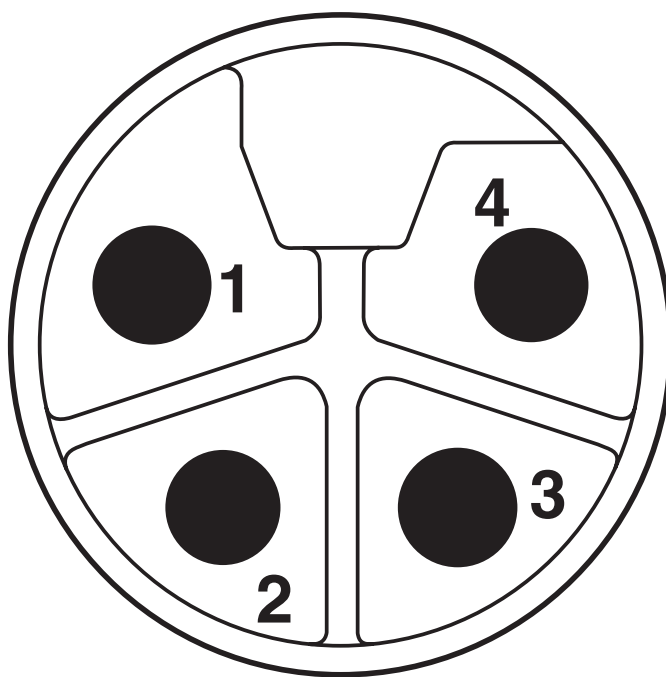
Układ styków wtyku M12, 4-pinowy, kodowanie L, widok strony męskiej
