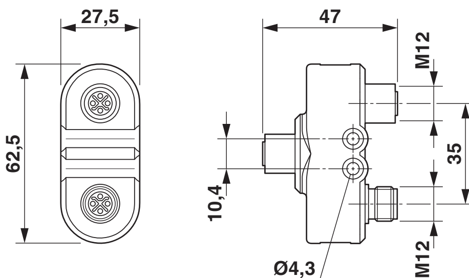
Rysunek wymiarowy
