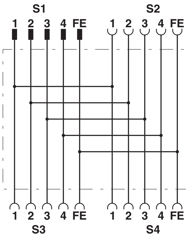
Schemat
