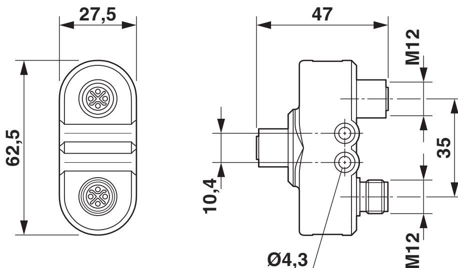
Rysunek wymiarowy
