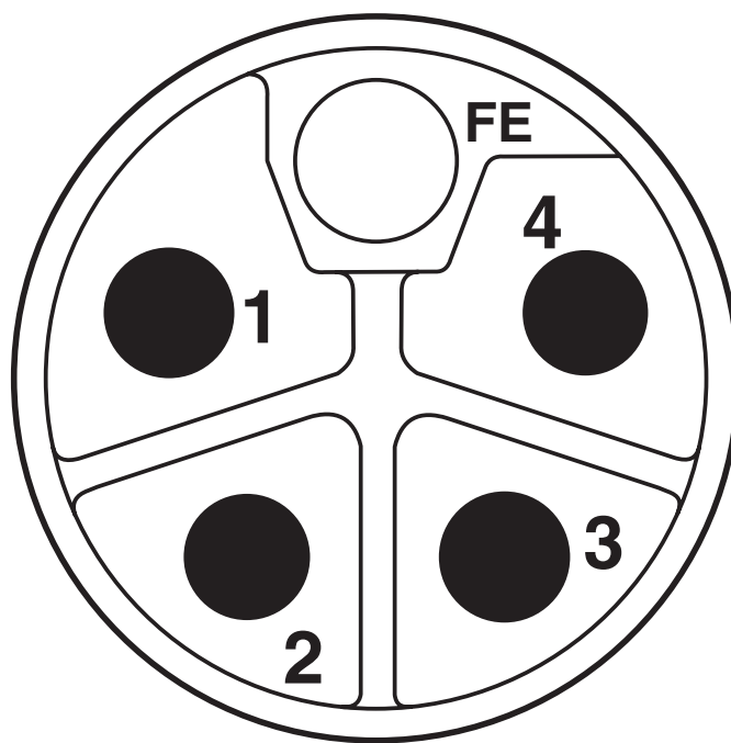
Układ styków wtyku M12, 5-pinowy, kodowanie L, widok strony męskiej
