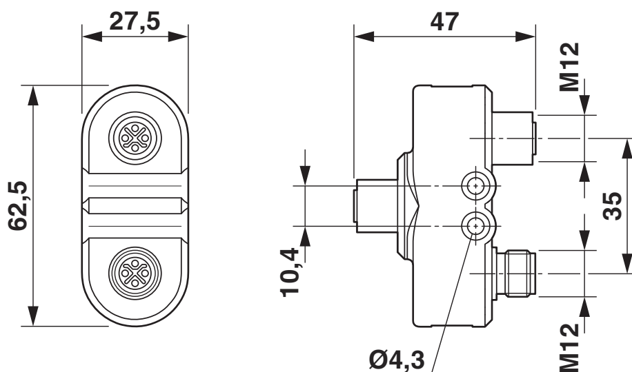
Rysunek wymiarowy
