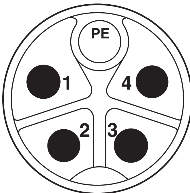
Układ styków wtyku M12, 4-bieg.+PE, kod. B, od strony wtyku
