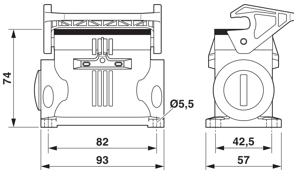
Rysunek wymiarowy
