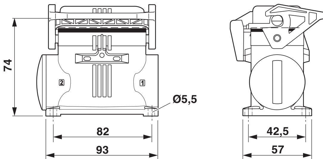
Rysunek wymiarowy
