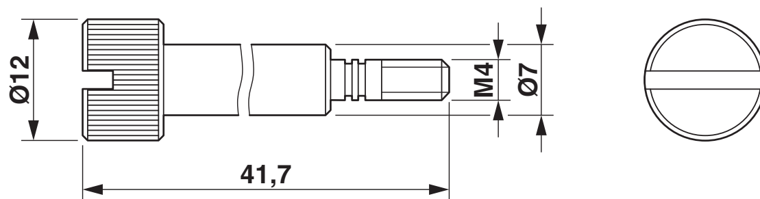
Rysunek wymiarowy
