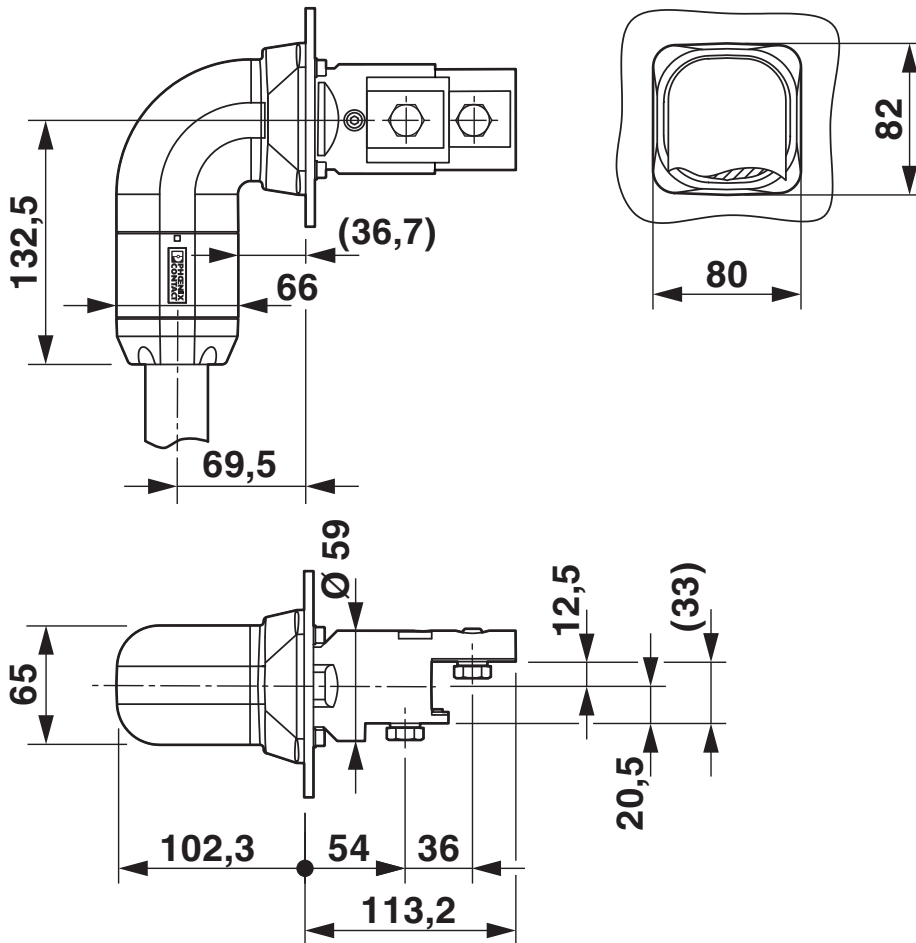
Rysunek wymiarowy
