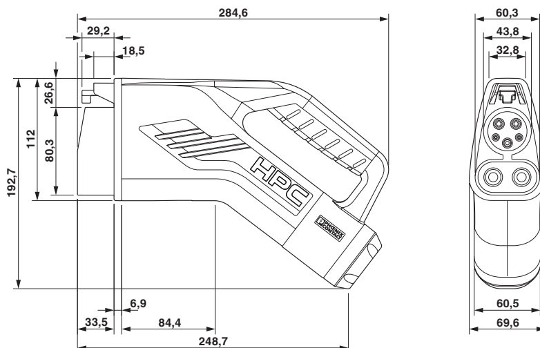
Rysunek wymiarowy
