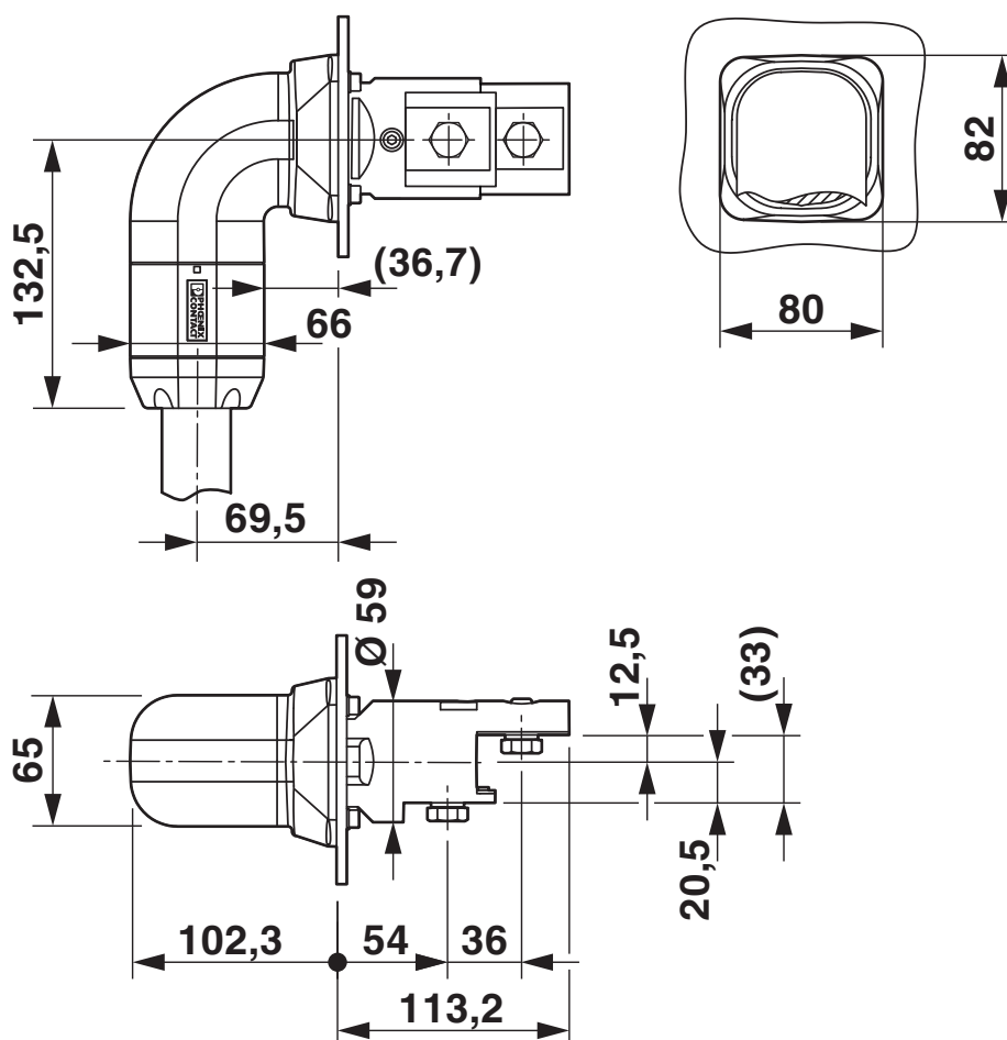
Rysunek wymiarowy
