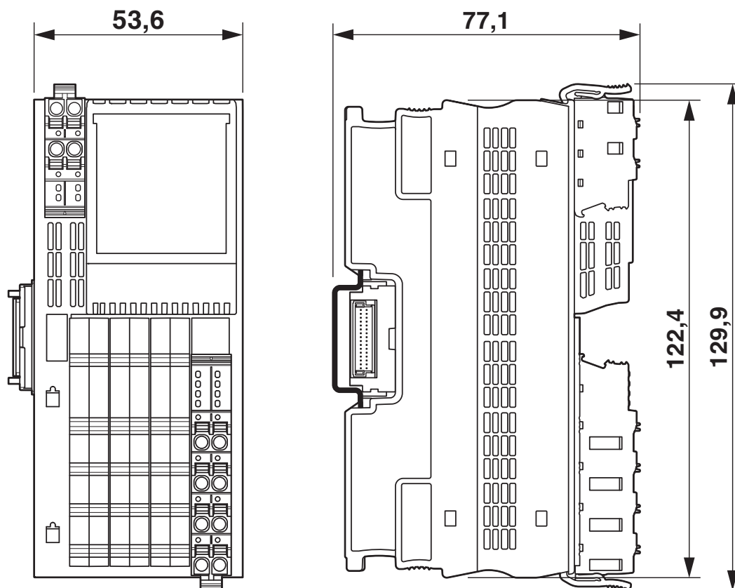
Rysunek wymiarowy
