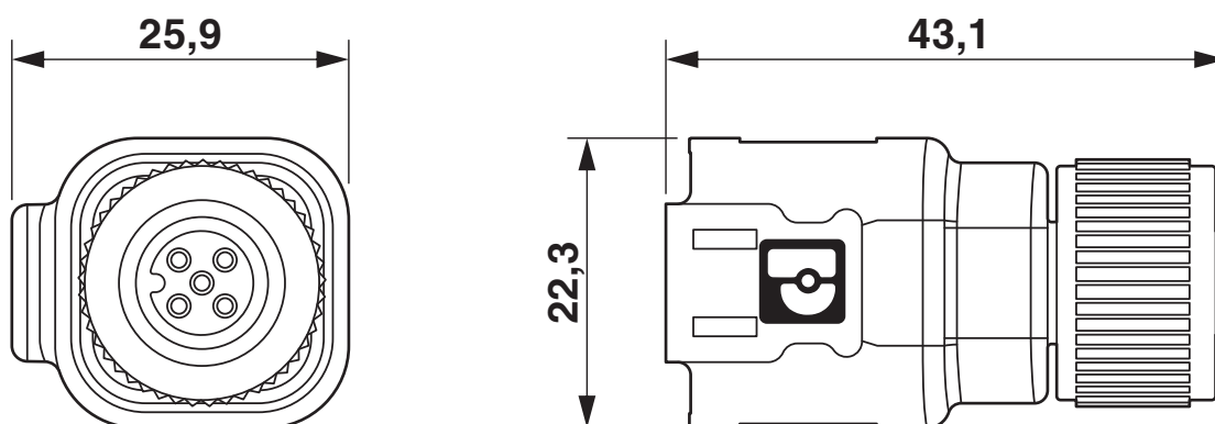
Rysunek wymiarowy
