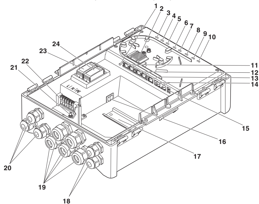
Rysunek schematyczny
