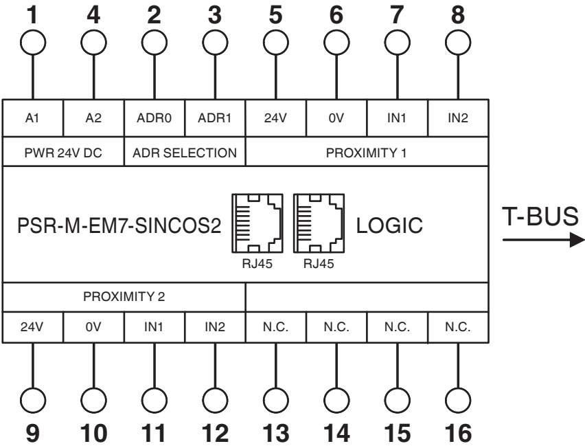
Schemat blokowy
