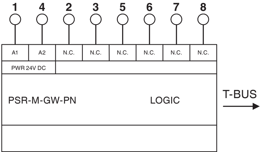
Schemat blokowy
