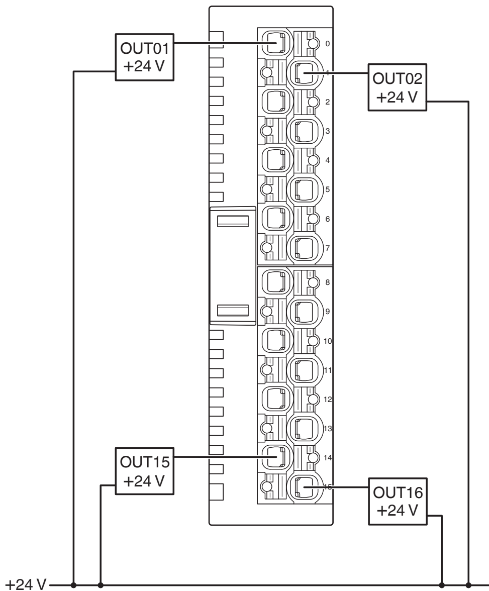
rysunek złączy
