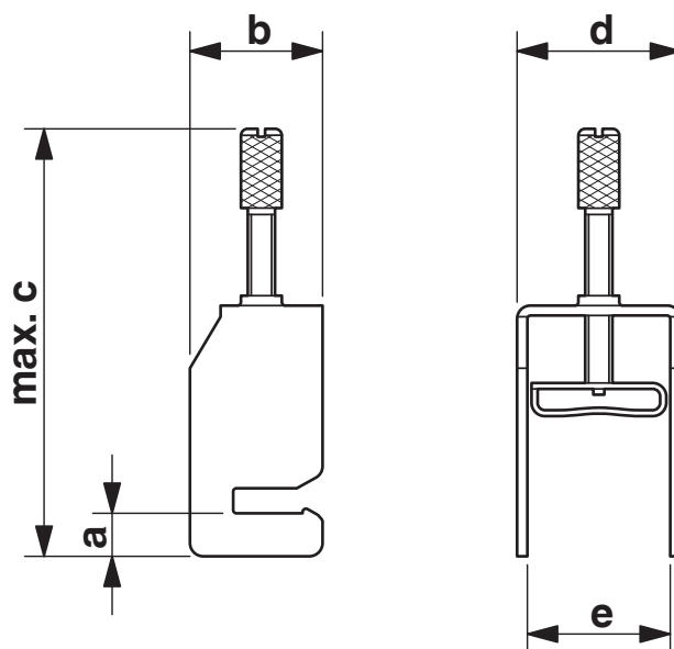
Rysunek wymiarowy
