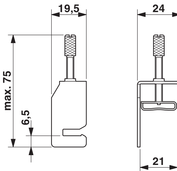
Rysunek wymiarowy
