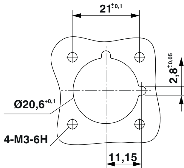
Rysunek wymiarowy
