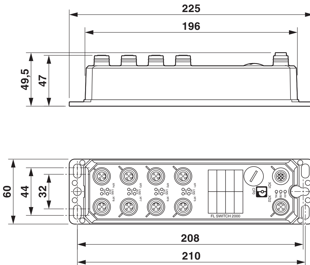
Rysunek wymiarowy
