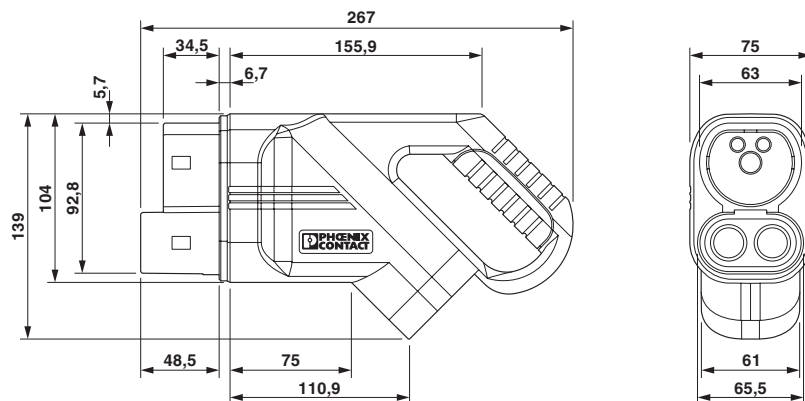
Rysunek wymiarowy
