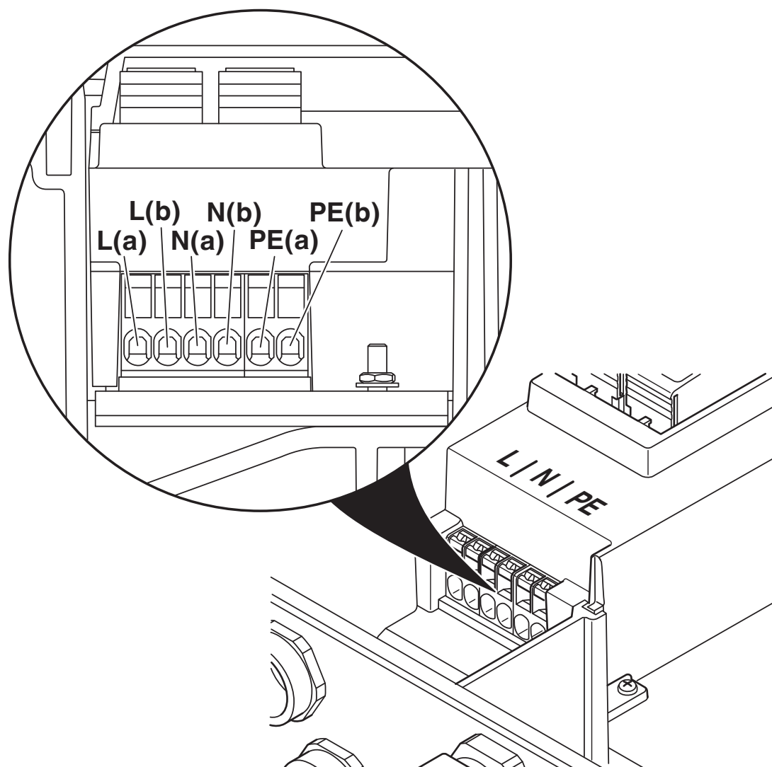
rysunek złączy
