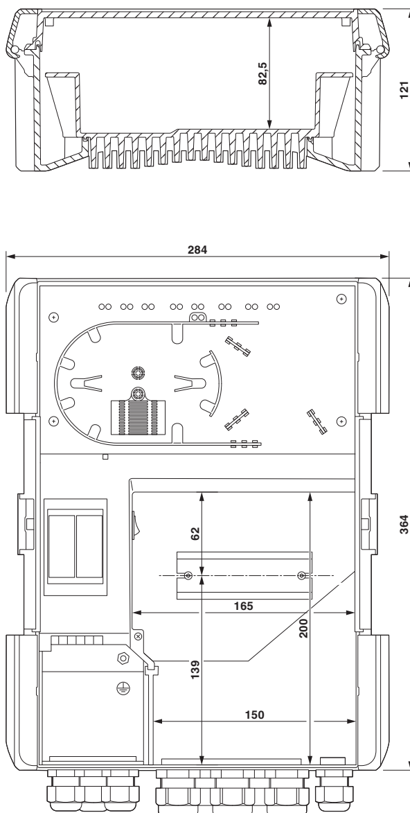
Rysunek wymiarowy
