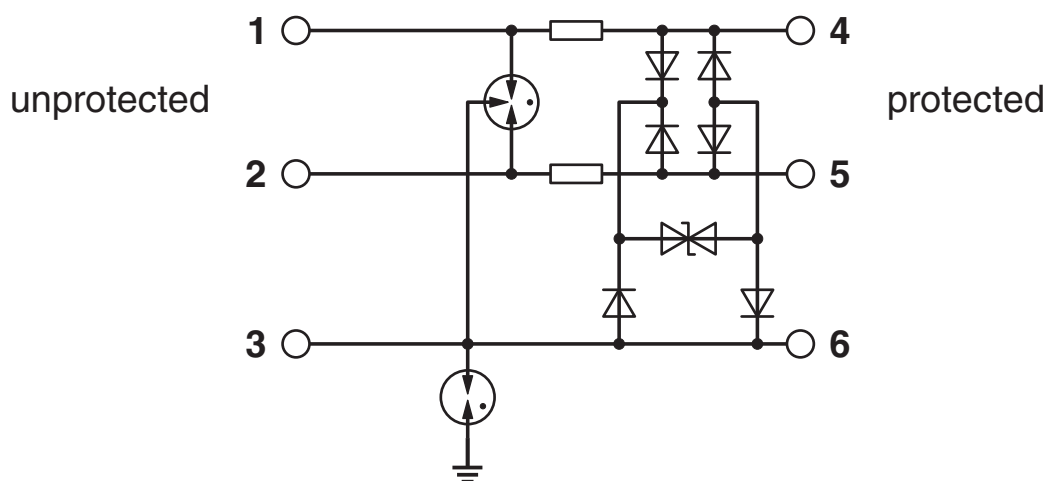
Schemat
