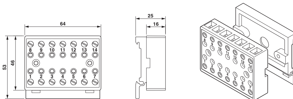
Rysunek wymiarowy
