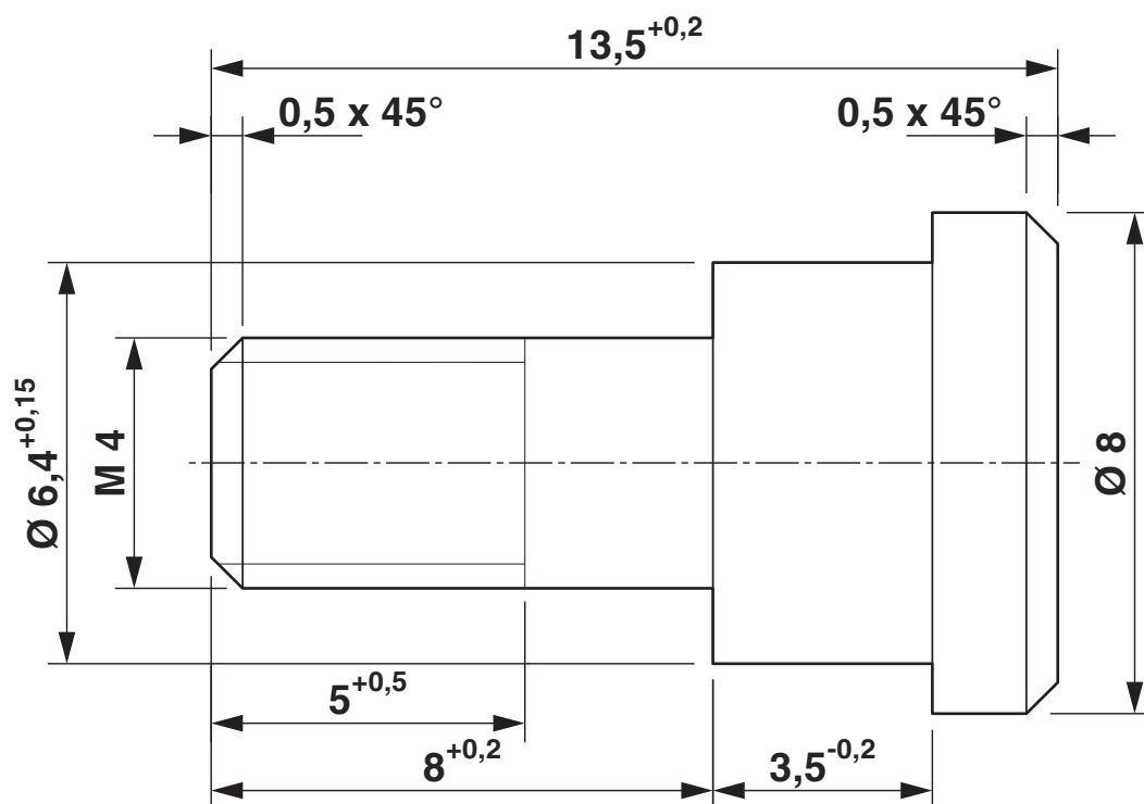
Rysunek wymiarowy
