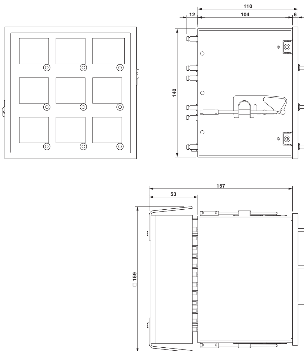
Rysunek wymiarowy
