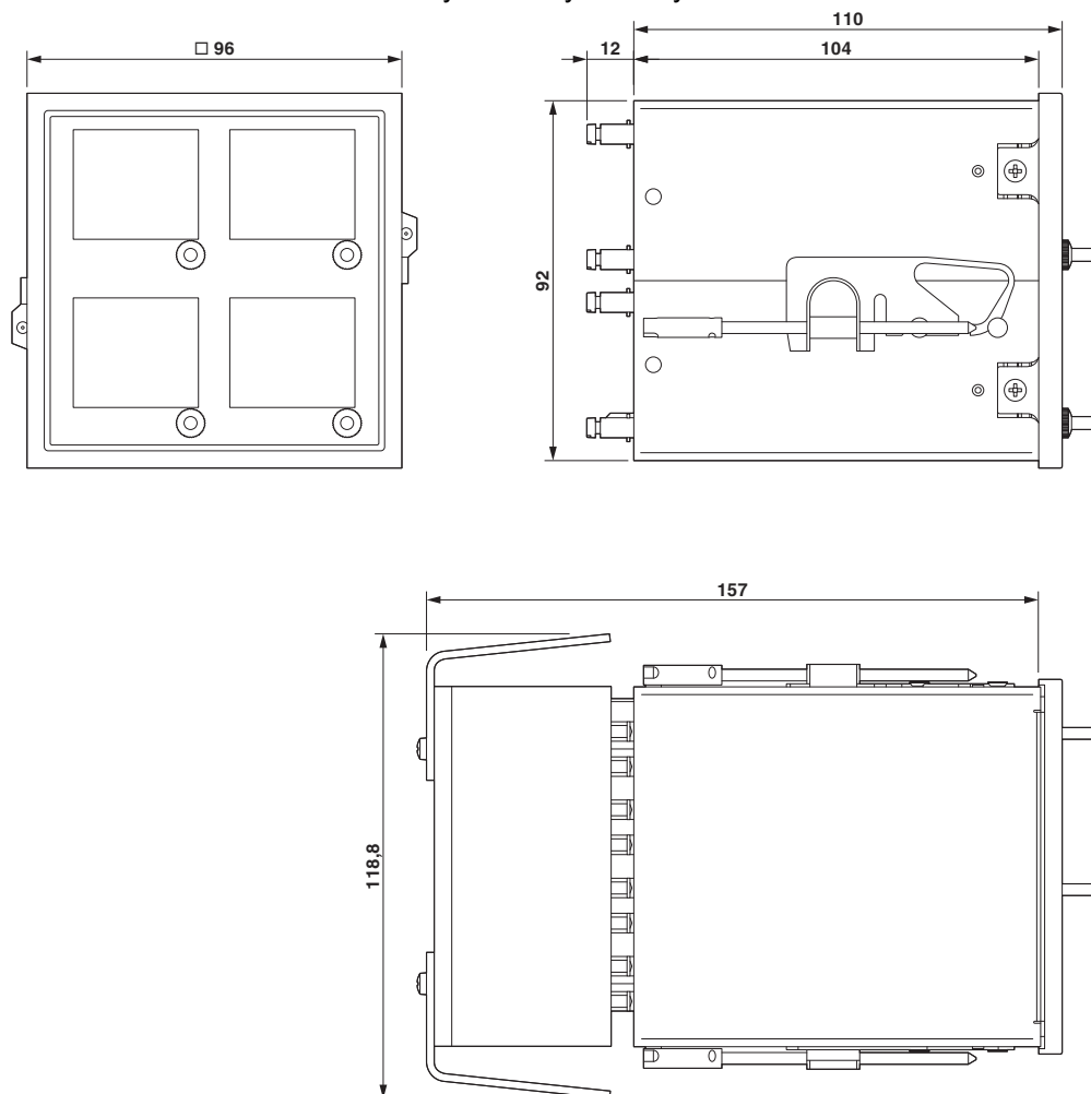
Rysunek wymiarowy
