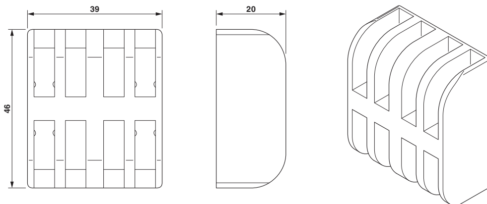
Rysunek wymiarowy
