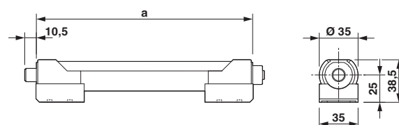
Rysunek wymiarowy
