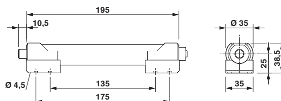
Rysunek wymiarowy
