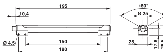
Rysunek wymiarowy
