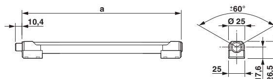
Rysunek wymiarowy
