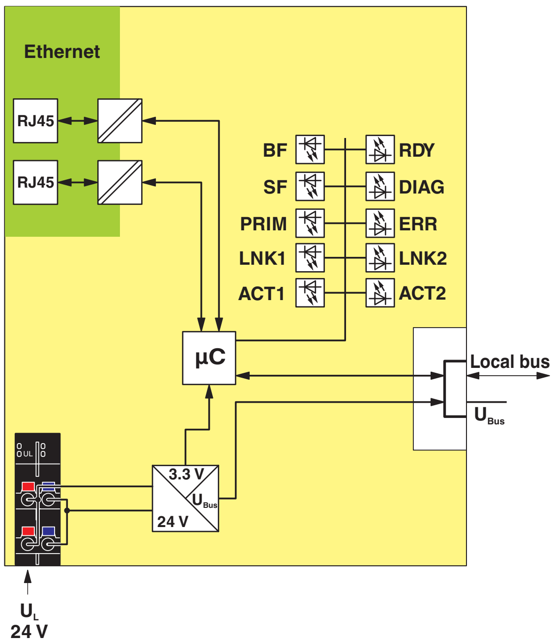
Schemat blokowy
