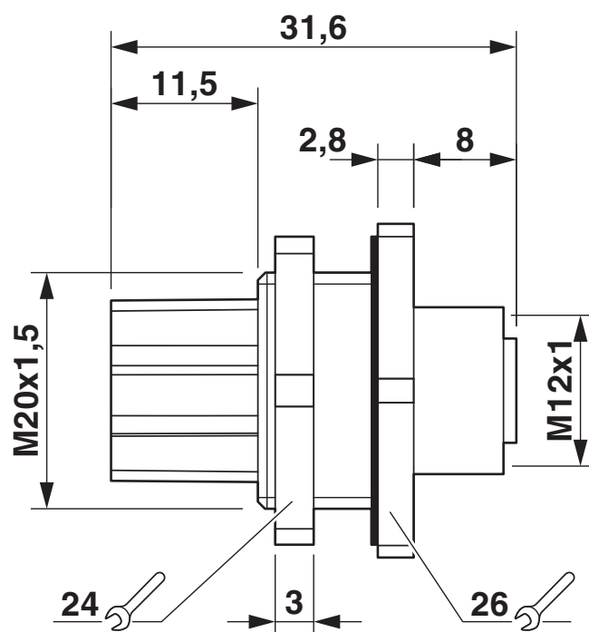
Rysunek wymiarowy
