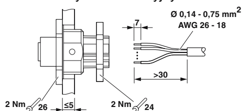
rysunek funkcyjny
