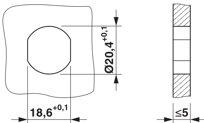
Otworowanie/geometria płytek lutowniczych
