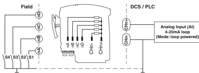
Rysunek schematyczny
