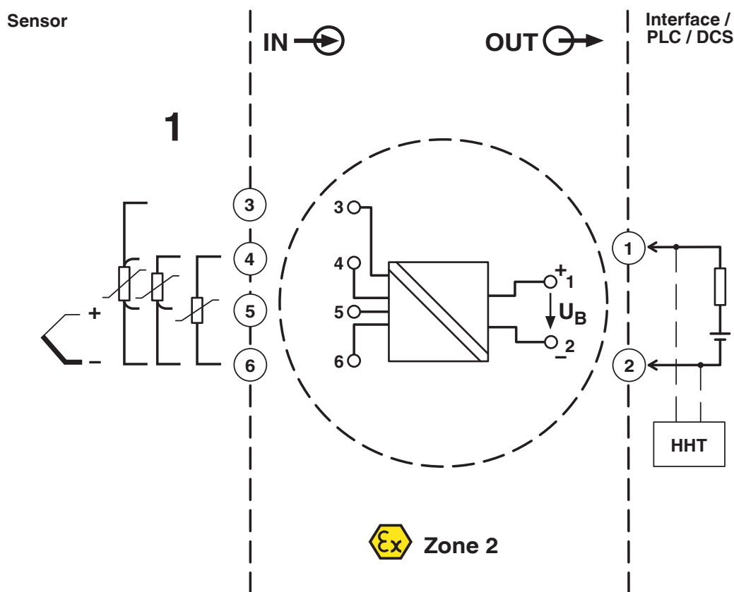
Schemat blokowy
