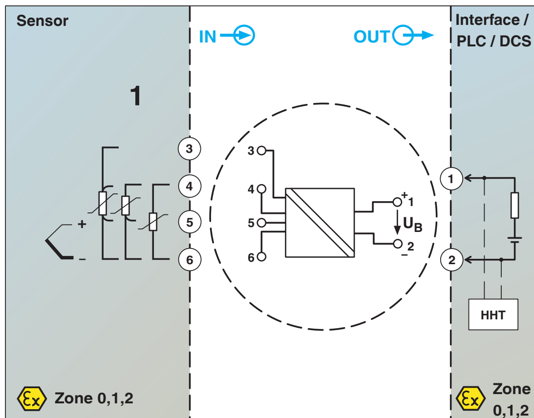
Schemat blokowy
