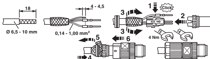
rysunek funkcyjny
