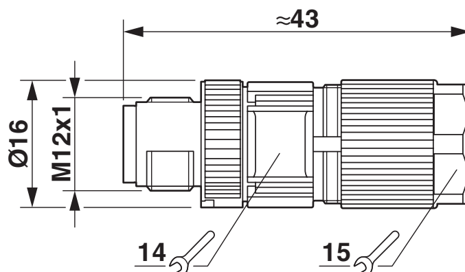
Rysunek wymiarowy
