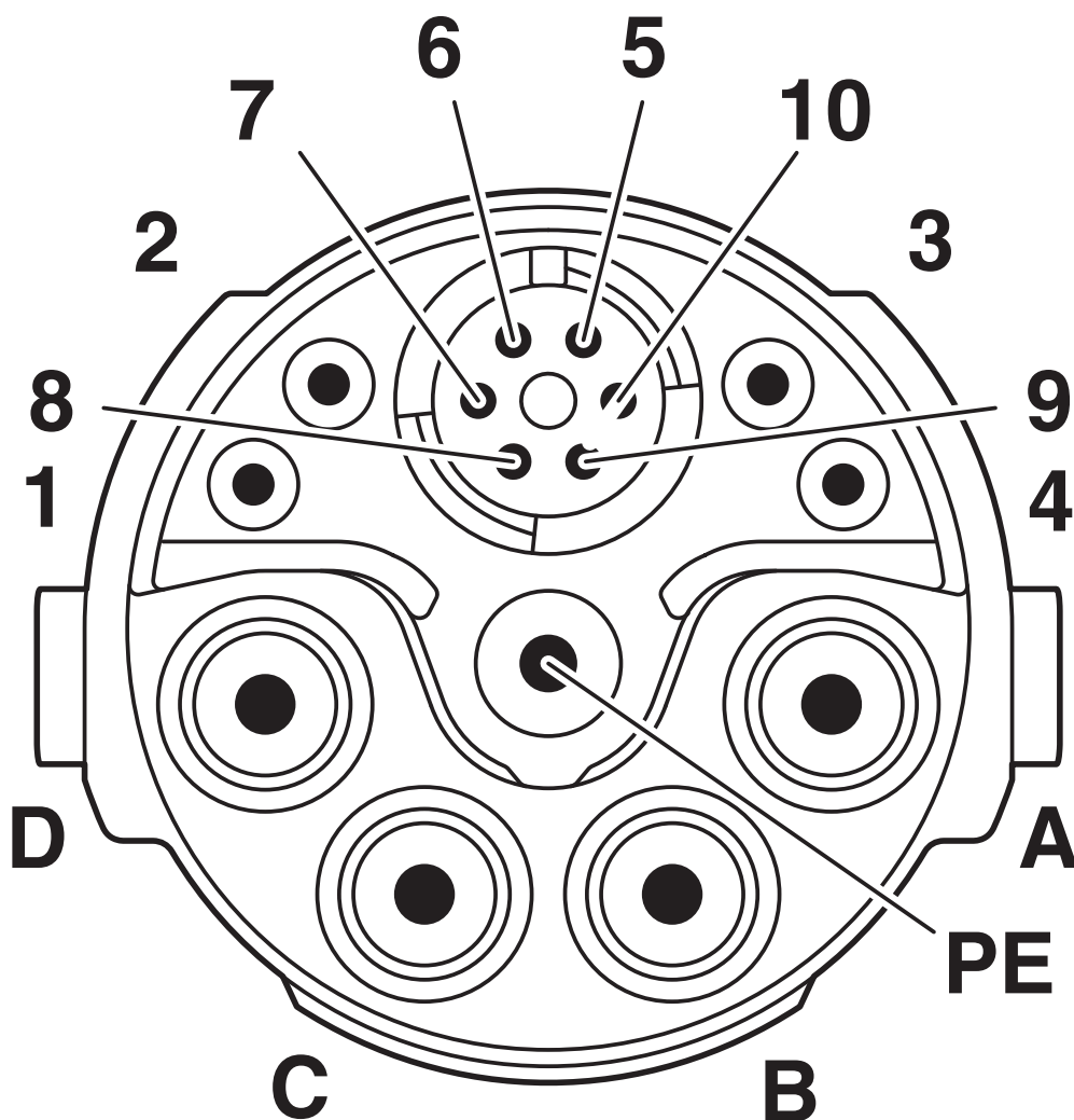
Rysunek schematyczny
