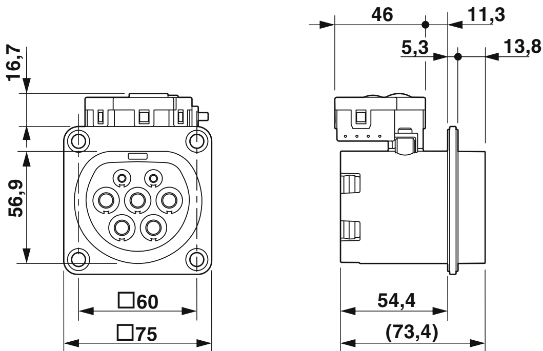
Rysunek wymiarowy
