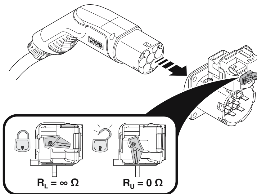
Rysunek schematyczny
