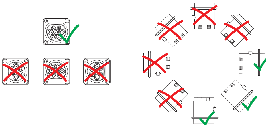
Rysunek schematyczny
