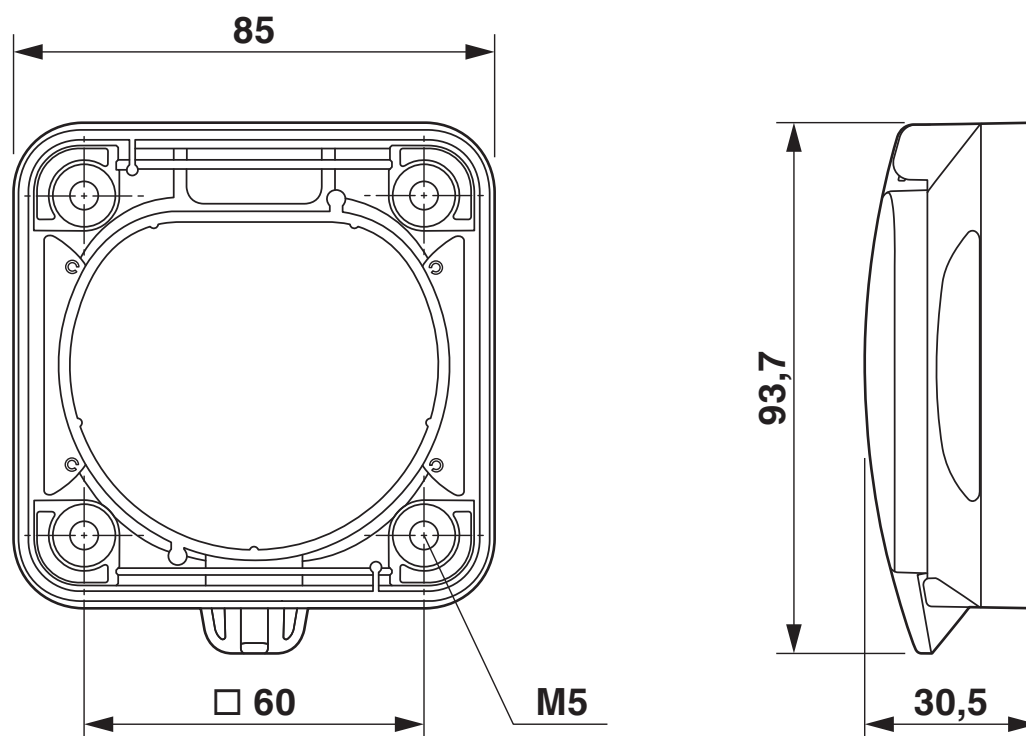
Rysunek wymiarowy
