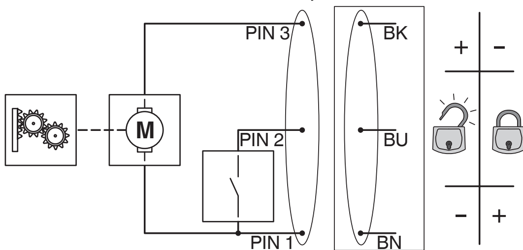
Schemat blokowy silownika blokady
