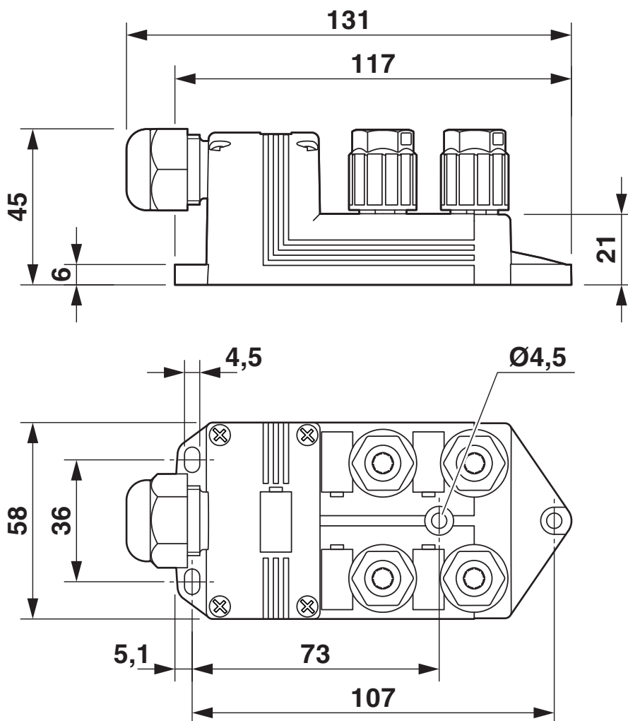
Rysunek wymiarowy
