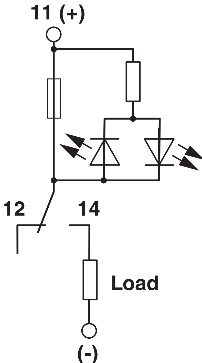
Schemat
