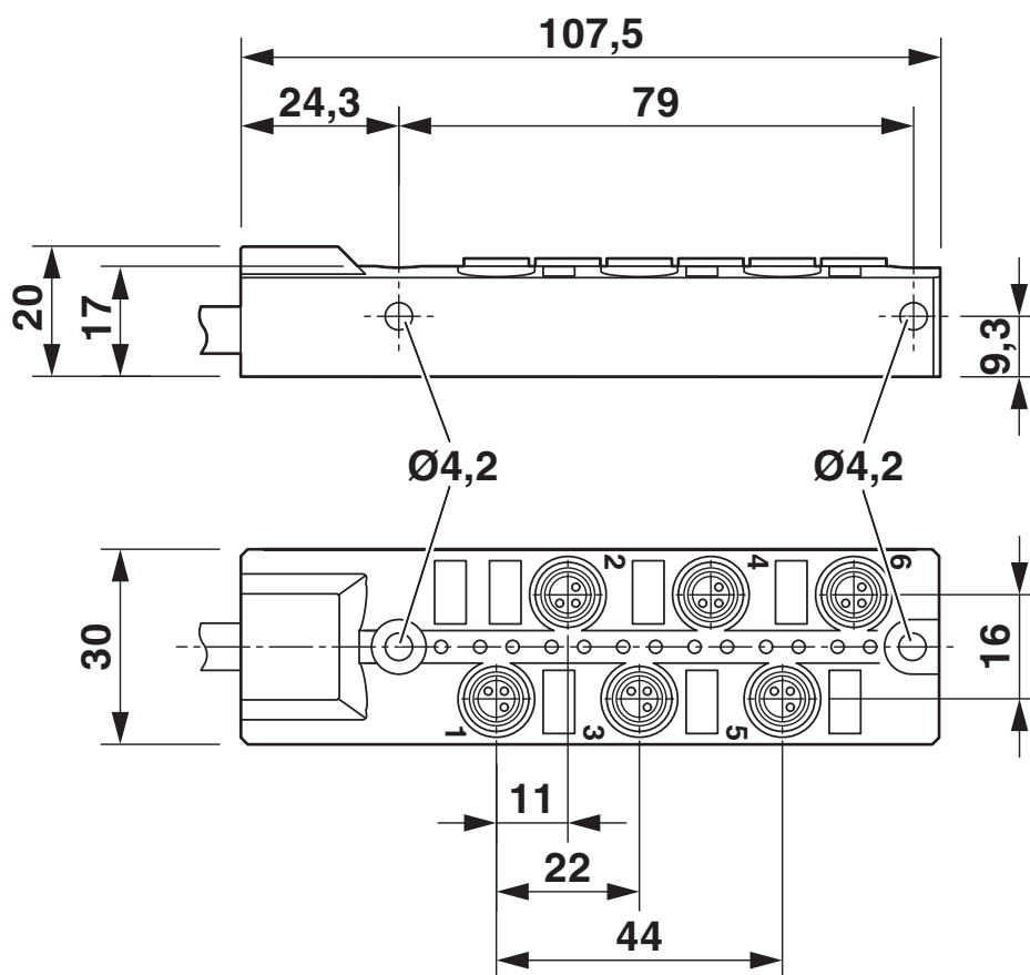
Rysunek wymiarowy
