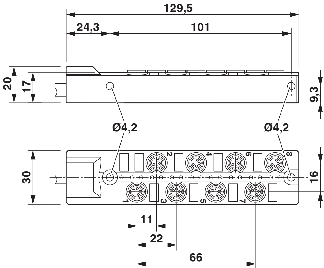
Rysunek wymiarowy
